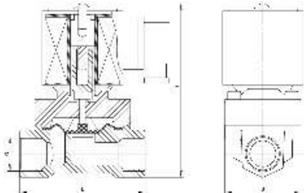
Рис. 2. Клапан тип VS
